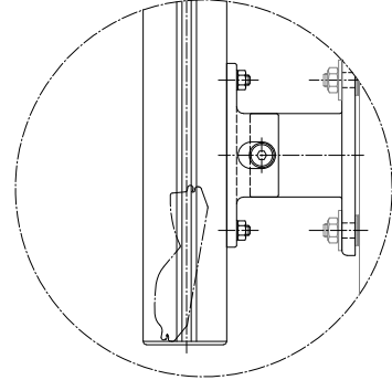
Detalje mørkelægningslamel
